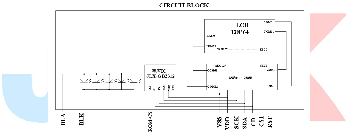
图 2: 电路框图
