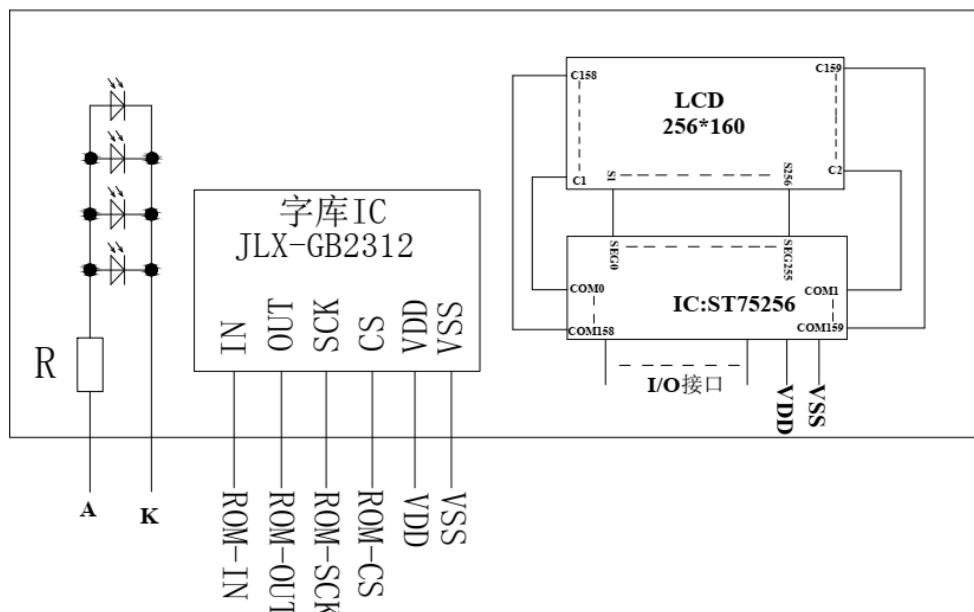
图 2: JLX256160G-9803-PL 电路框图
