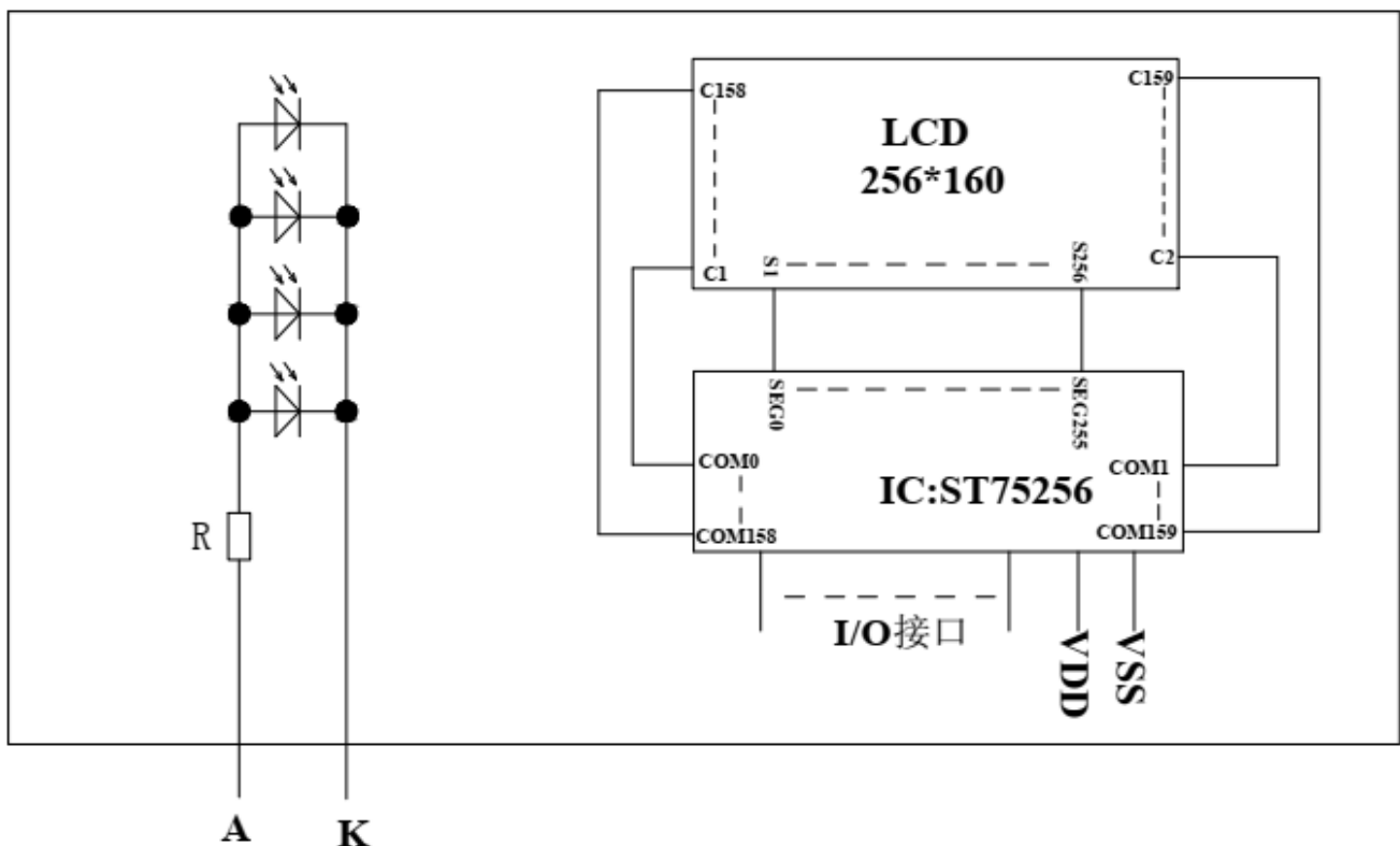
图 2: JLX256160G-9803-PN 图像点阵型液晶模块的电路框图
