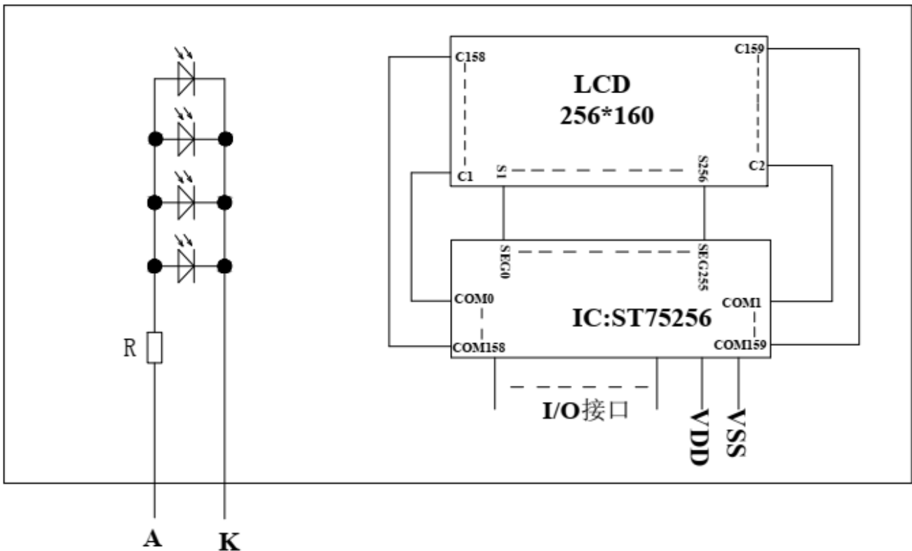
图 2: JLX256160G-9803-BN 图像点阵型液晶模块的电路框图
