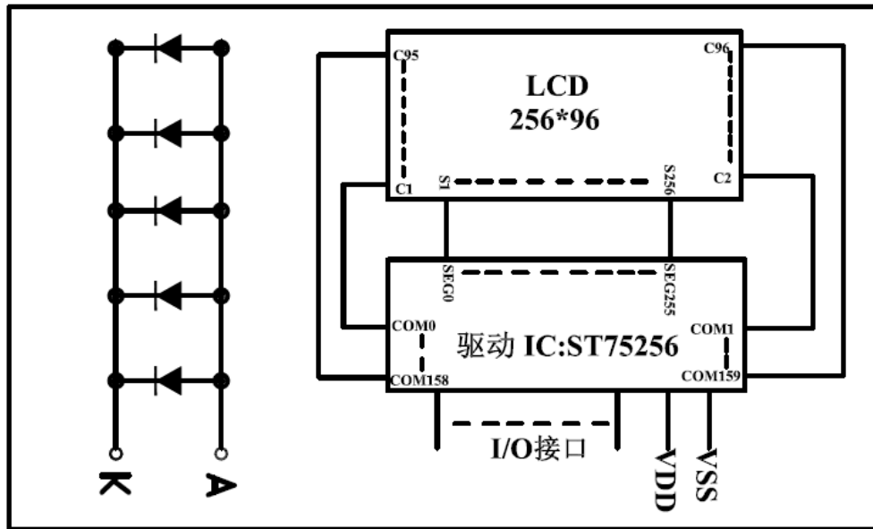
图 2: JLX25696G-968-BN 图像点阵型液晶模块的电路框图
